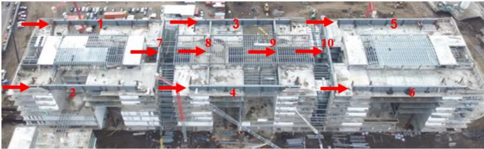
Figura 16a Vista aérea de las 10 vigas-puente alojadas en último piso de la Plataforma Gubernamental Social durante la etapa de construcción de la estructura.
