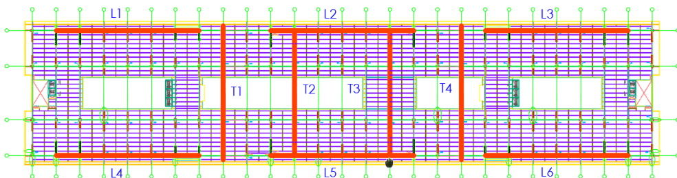
Figura 14. Arreglo reticular ubicado en el último piso de la Plataforma Social, el peso conjunto de estas 10 vigas corresponde a 700 toneladas de acero estructural. (L: Longitudinal; T: Transversal).
