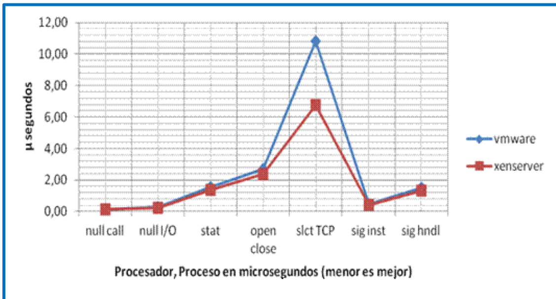
Figura 2. Evaluación del Procesador mediante Lmbench
