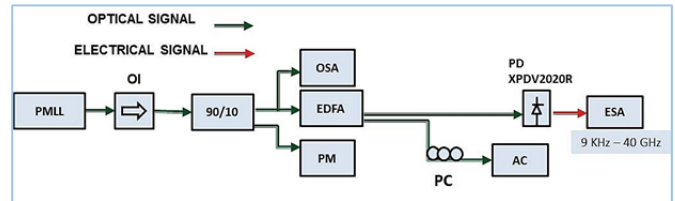
Fig. 13. Setup experimental. PMLL: láser modelocked pasivo. OI: Aislador Optico. OSA: Analizador de Espectro Optico. EDFA: Amplificador de fibra dopada de erbio. PM: medidor de potencia. PC: control de polarización. AC: autocorrelador. PD: fotodiodo modelo XPDV2020R. ESA: Analizador de Espectros Eléctrico.
