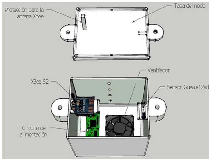
Fig. 6. Diseño de la estructura del nodo 2.
