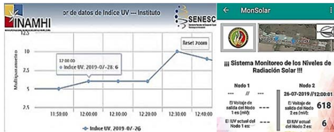
Fig. 18. Gráfica del IUV obtenido, entre INAMHI y el sensor GUA- S12SD, en función de tres de las horas (11-12-13 horas) con mayor radiación en el día (clima: soleado y semi-templado).
