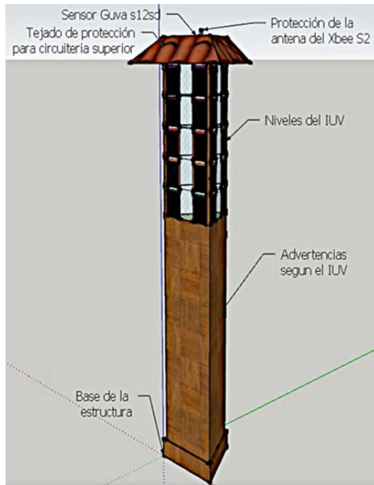
Fig. 7. Diseño de la estructura del solmáforo.
