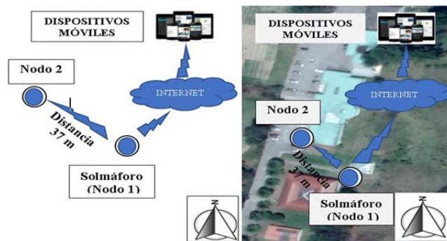
Fig. 5. Arquitectura del Sistema de monitoreo establecido.
