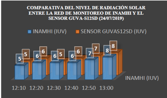
Fig. 15. Gráfica del IUV obtenido, entre INAMHI y el sensor GUYA-S12SD, en función de las 12 horas del día (clima: soleado y nublado).
