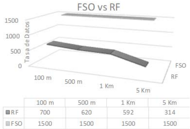
Fig. 18. Comparativa entre FSO y RF en cuanto a transmisión de tasa de bits
