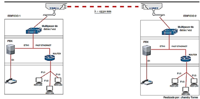
Fig. 2. Diagrama de red FSO
