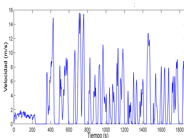
Fig. 3. Velocidad del ciclo de conducción BADC
