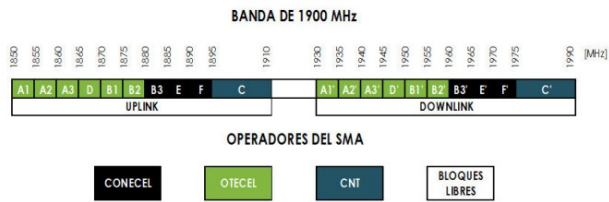
Fig. 5. Asignación de espectro SMA según ARCOTEL
