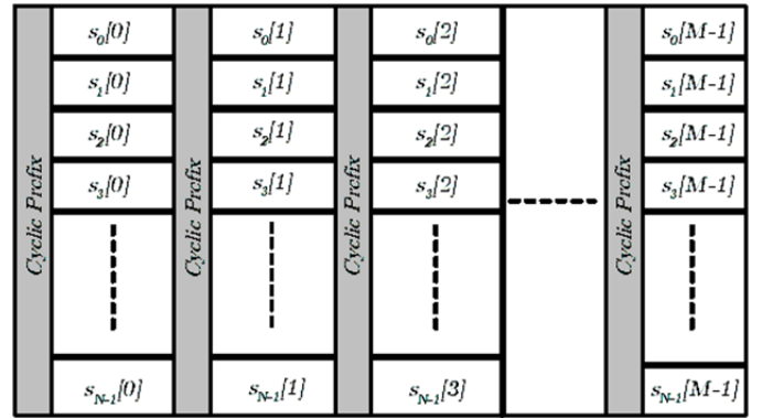
Fig. 4. Paquete de datos del sistema OFDM.
