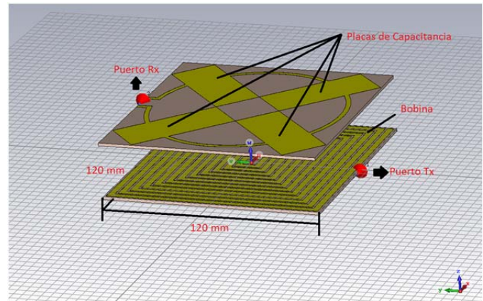
Fig. 2. Alineación de la antena transmisora y receptora separadas por el espacio libre
