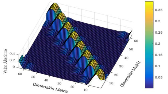
Fig. 8. Matriz de transmisión \mathbf{Y} GFDM.
