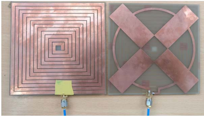
Fig. 11. Antenas impresas en el sustrato FR4
