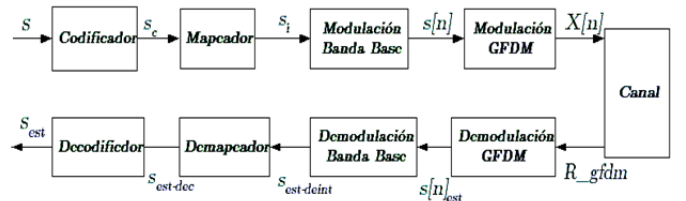
Fig. 5. Diagrama en bloque del sistema GFDM.
