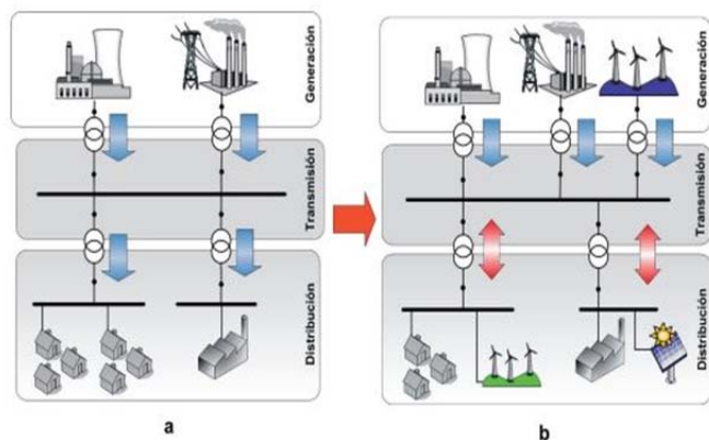
Fig. 1. Sistemas de energía eléctrica (a) tradicional y (b) próxima generación [11]
