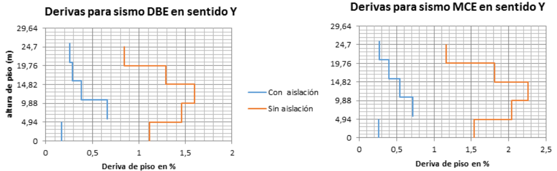
Figura 15 Derivas de Piso en Centro de Masa, para sismo actuando en sentido Y. Considerando estructura sin y con aisladores sísmicos.
