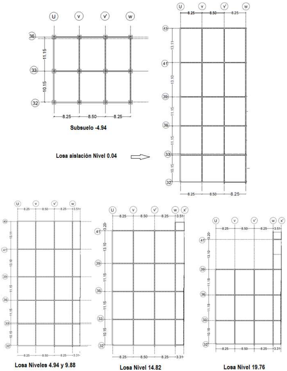
Figura 1 Plantas del Bloque Estructural 67 de la UFA-ESPE.
