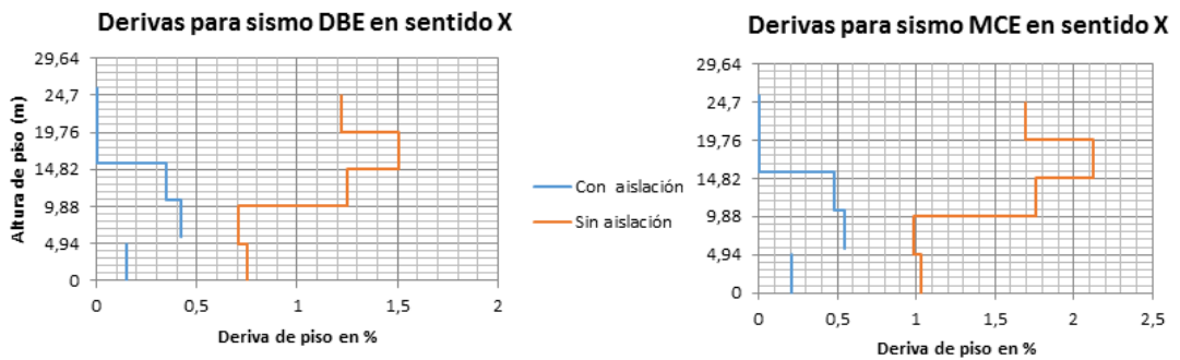
Figura 14 Derivas de Piso en Centro de Masa, para sismo actuando en sentido X. Considerando estructura sin y con aisladores sísmicos.
