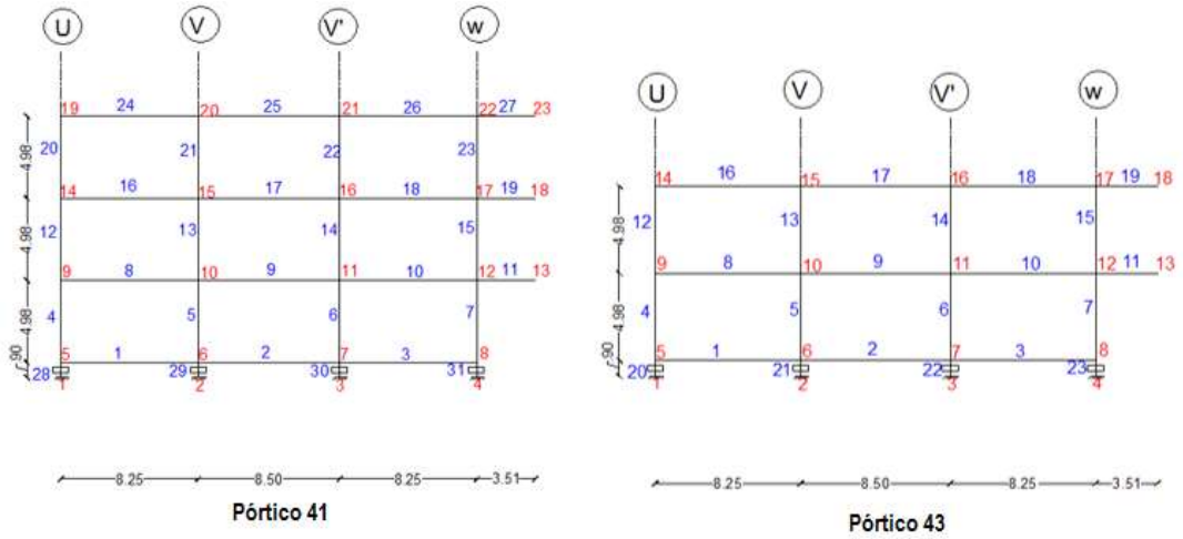
Figura 7 Pórticos en sentido X del Bloque Estructural 67
